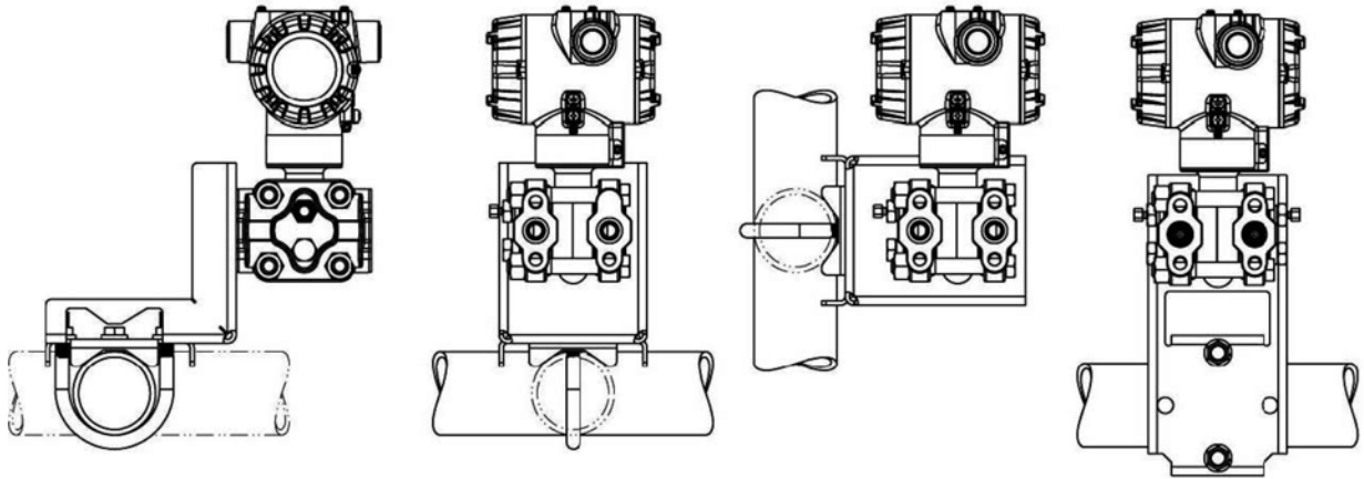
安装图
