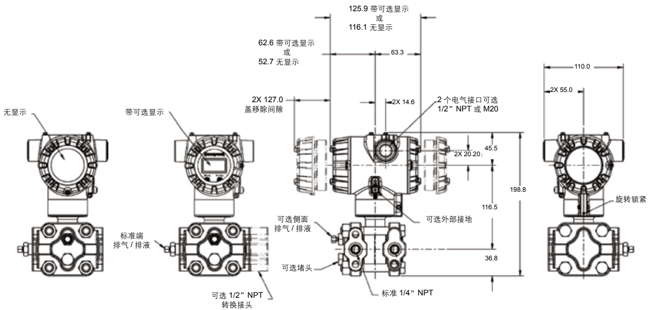
尺寸图
